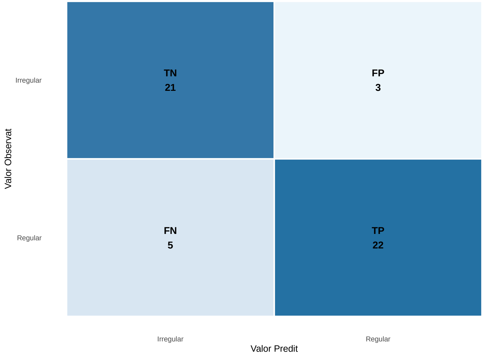
Matriu de confusió — CatBoost (validació) Llindar = 0.515 | Precision = 0.8800 | Recall = 0.8148
